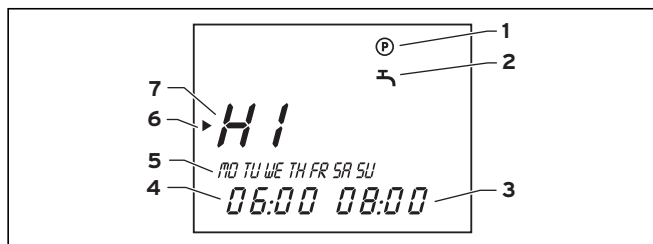
Fig. 4.7 Display programmeringsniveau
