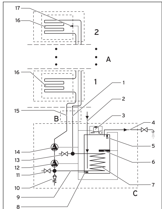
Fig. 2.3 Hovedkomponenter system auroSTEP plus med beholder VEH SN 250/3 i (principskitse uden tilslutnings-tilbehør)
