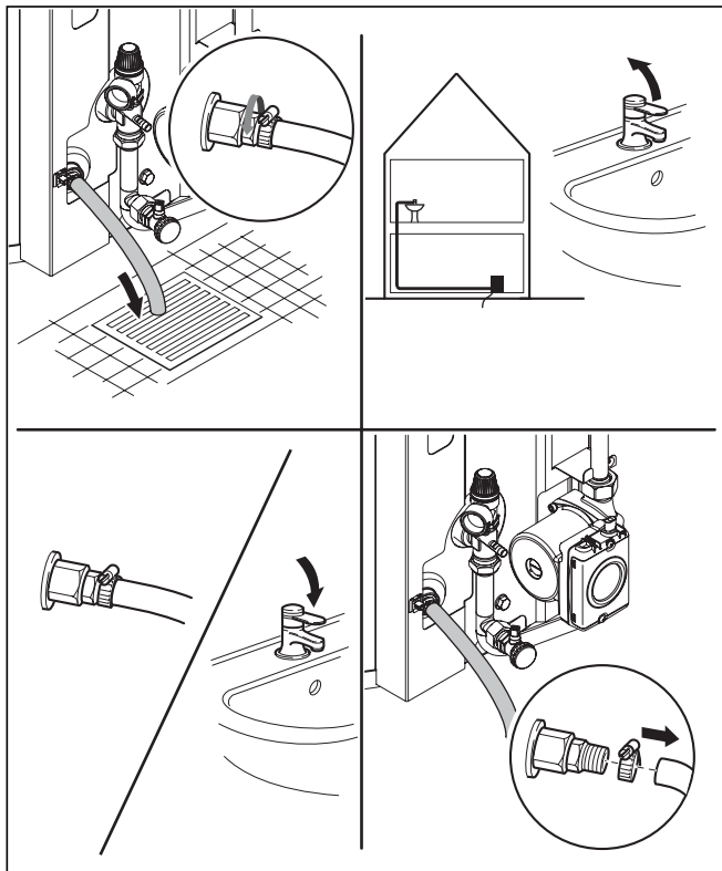
Fig. 4.8 Beholder tømmes
