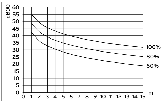
Fig. 6.4 Støjniveau fra to udeenheder i dB(A) afhængigt af afstand og ventilatorens omdrejningstal VWL 141/3 S ved opstilling i det fri
