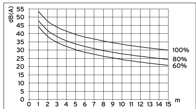
Fig. 6.2 Støjniveau fra en udeenhed i dB(A) afhængigt af afstand og ventilatorens omdrejningstal til VWL 81/3 S ved opstilling i det fri
