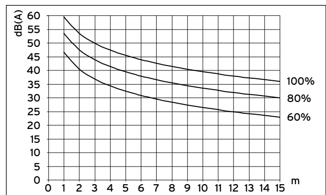
Fig. 6.3 Støjniveau fra en udeenhed i dB(A) afhængigt af afstand og ventilatorens omdrejningstal til VWL 101/3 S ved opstilling i det fri
