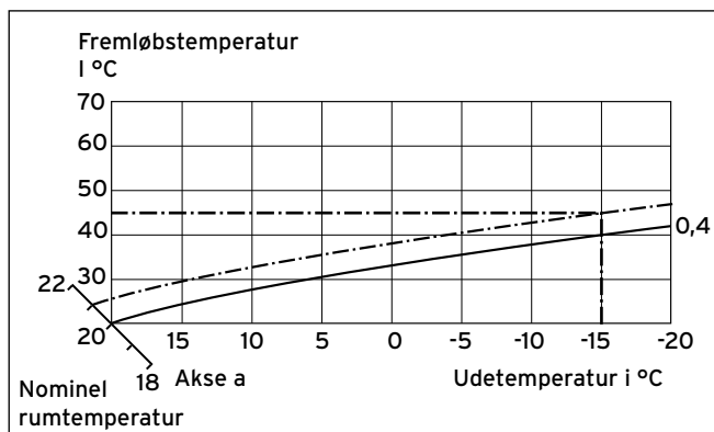
Fig. 2 Parallelforskydning af varmekurven
