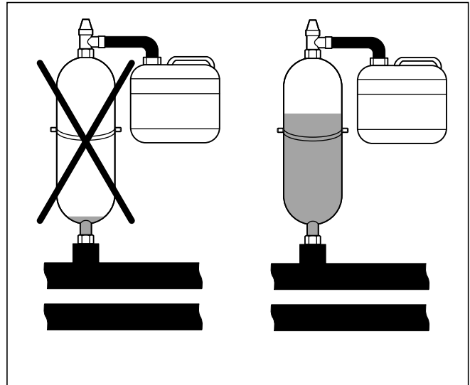
Fig. 6.6 Påfyldningsniveauet i brineekspansionsbeholderen
