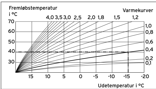
10.1 Diagram varmekurver
