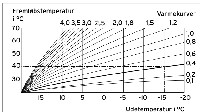
10.1 Diagram varmekurver
