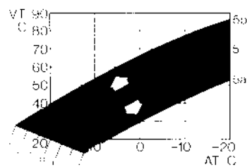
Indstillingsområde dagtemp.
