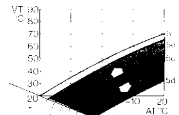
Indstillingsområde nattemp.
